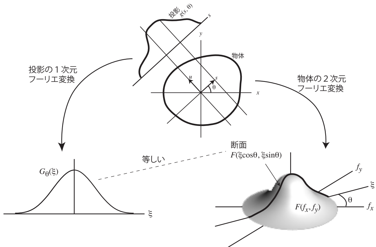
図 1: 投影定理.
