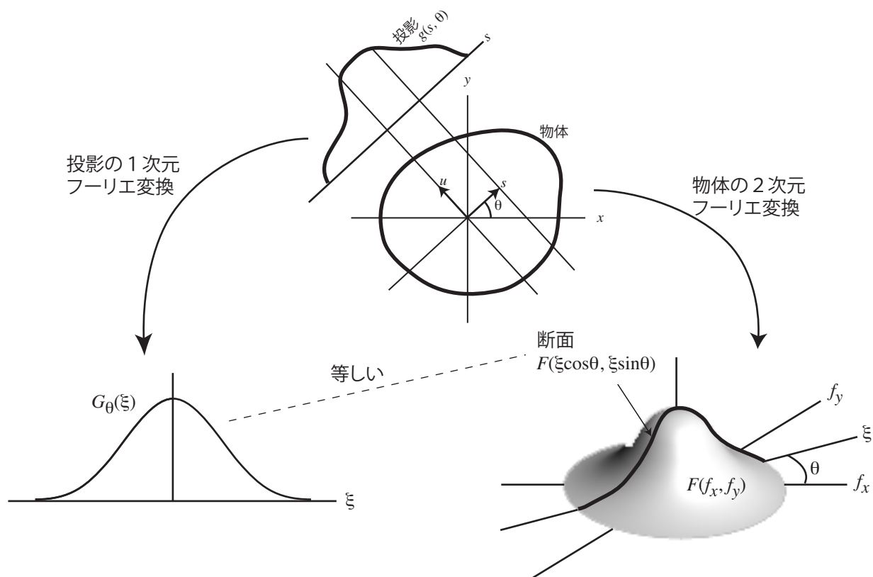
図 1: 投影定理.
